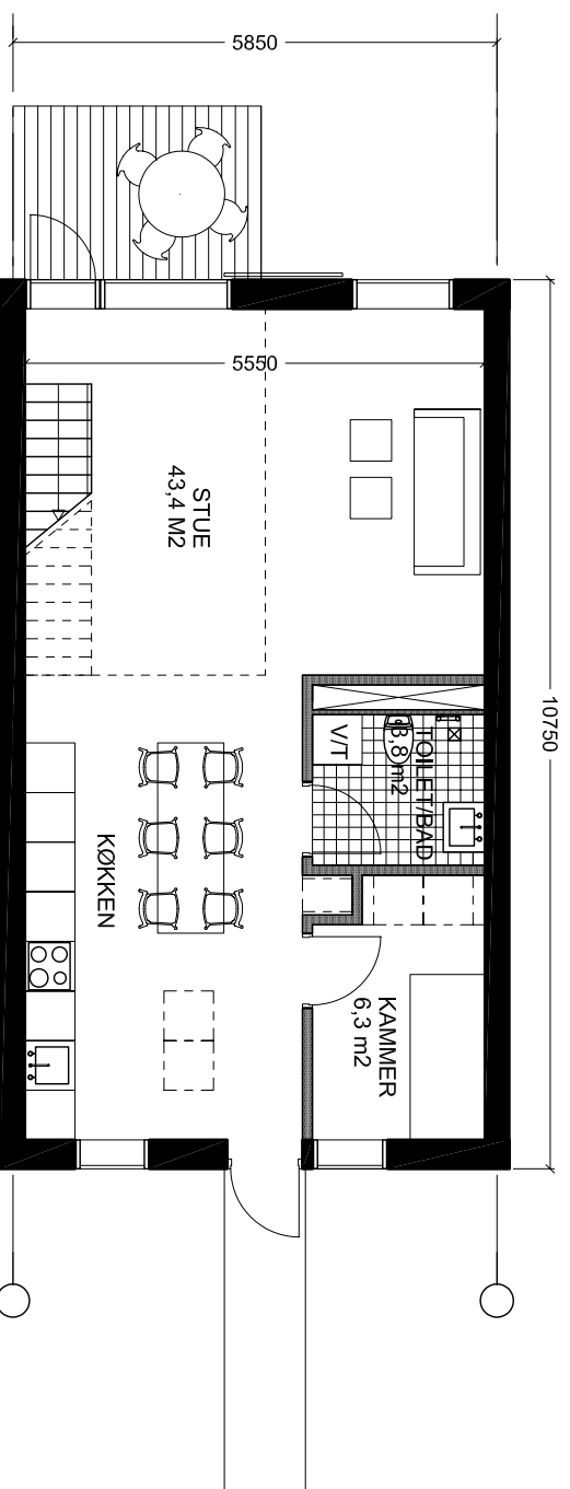
STUEPLAN LEJLIGHED C2 BRUTTO 63 M2 TOTAL: 115 M2 3 VÆRELSE 1 KAMMER
