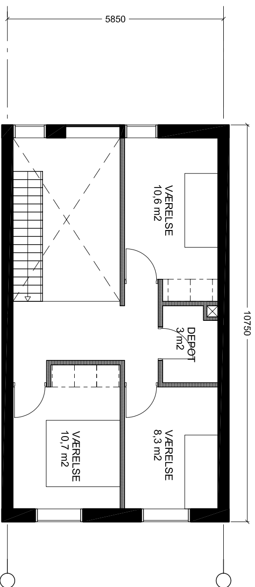
1. SALS PLAN LEJLIGHED C2 BRUTTO 52 M2
